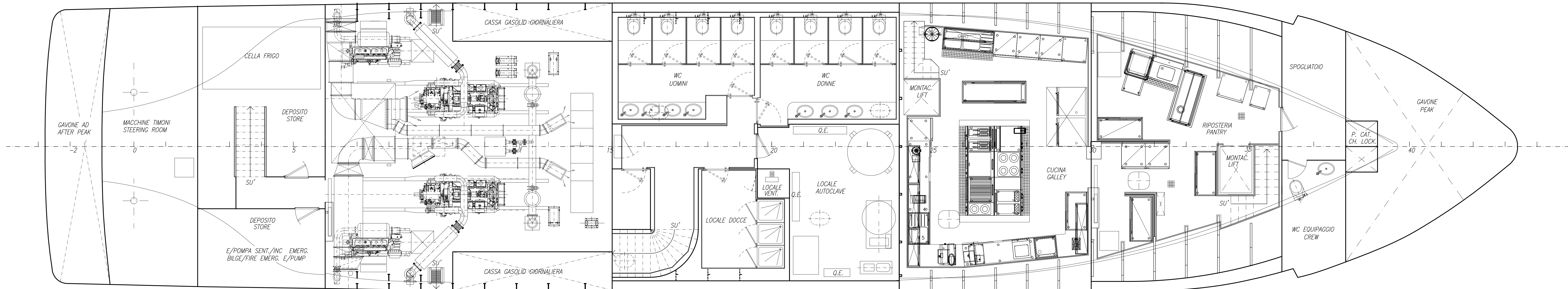
PIANO DI STIVA TANK TOP
