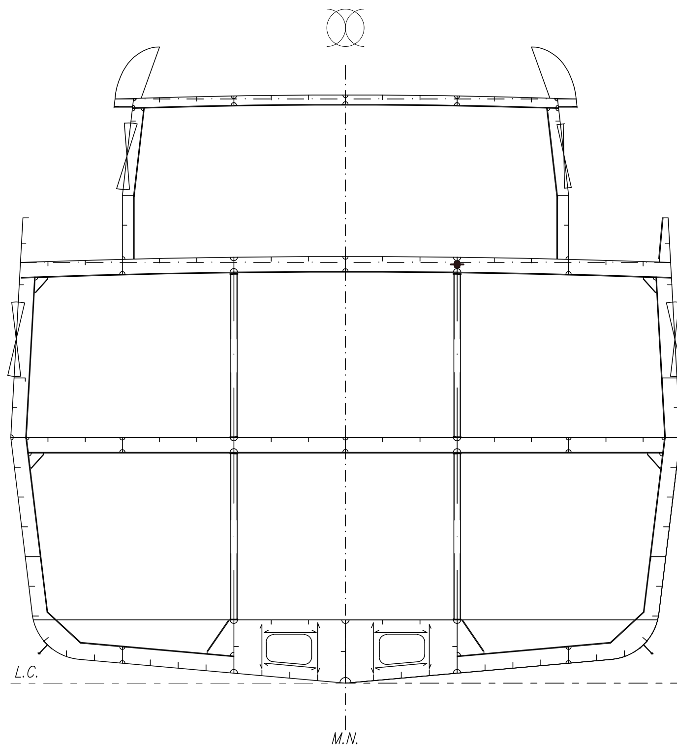
SEZIONE MAESTRA MIDSHIP SECTION
